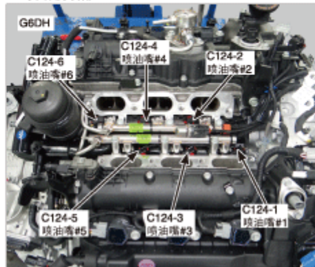
26. 发动机顶部
