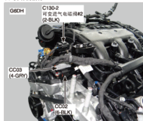
30. 发动机前部
