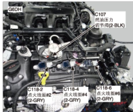
25. 发动机左侧
