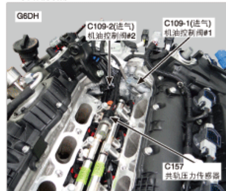
27. 发动机顶部
