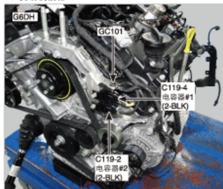
29. 发动机前部
